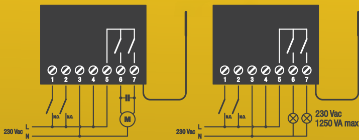
branchements pour la commande d'un moteur
